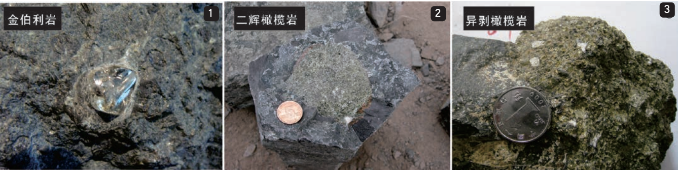
1 为山东蒙阴地区含有金刚石的古生代金伯利岩，2 和 3 为山东昌乐地区含有地幔橄榄岩包体的新生代玄武岩。金伯利岩是金刚石的母岩，而天然金刚石形成于地下大约 180 千米的深度。对金伯利岩的研究表明，华北克拉通破坏之前岩石圈的厚度大约有 200 千米。而对新生代玄武岩携带的地幔橄榄岩包体的研究表明，华北克拉通东部岩石圈的厚度在新生代仅有 60 ~ 80 千米。也就是说，中生代以来，华北克拉通东部岩石圈厚度减薄了上百千米。
