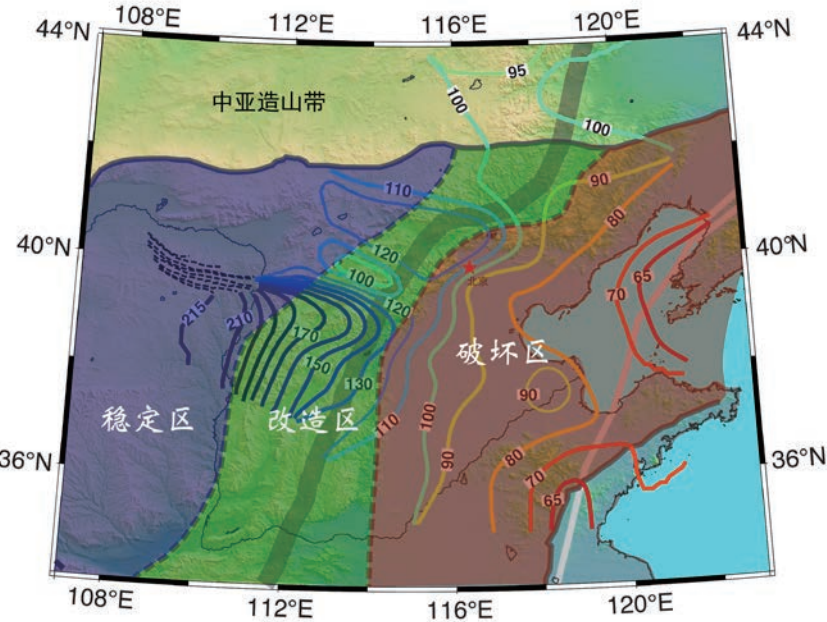
地震探测获得的华北克拉通岩石圈厚度分布 朱日祥提出以流动地震台阵探测华北克拉通深部结构的研究思路，通过大规模天然地震观测，获得了华北克拉通岩石圈的高分辨率结构信息。发现了东部陆块岩石圈（厚约 60 ~ 100 千米）明显不同于典型克拉通型岩石圈结构，西部陆块岩石圈（厚达 210 千米）则保持典型克拉通的特征，而中部陆块地壳则介于东部和西部之间。图中等值线（单位为千米）表示岩石圈的厚度。
