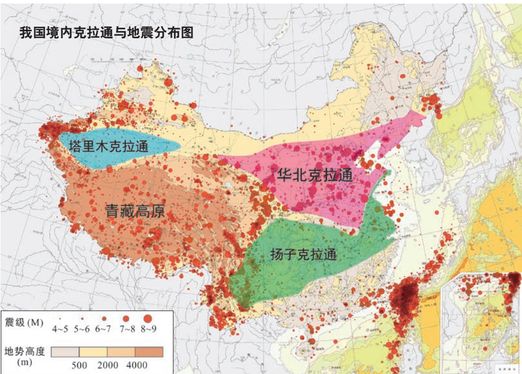
我国境内的 3 个克拉通包括从甘肃陕西到辽宁和朝鲜半岛的华北克拉通，从我国西南到长江中下游的扬子克拉通，以及新疆的塔里木克拉通。从图中可以明显看到，相比于扬子克拉通和塔里木克拉通，华北克拉通内部发生了数量更多的地震（包括 1976 年造成 24 万余人丧生的唐山大地震），这表明华北克拉通失去了稳定性。
